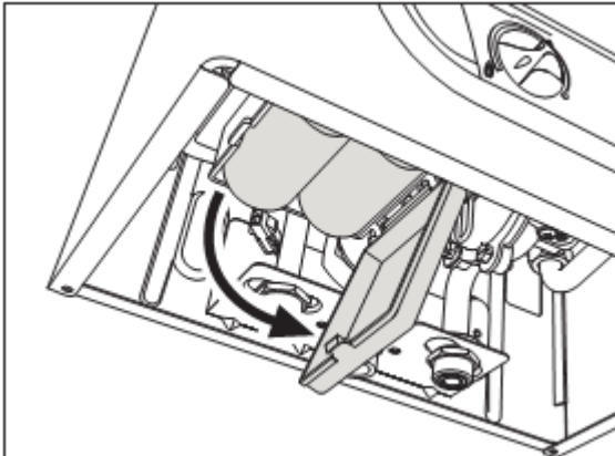
fig. 12 De batterijen vervangen
