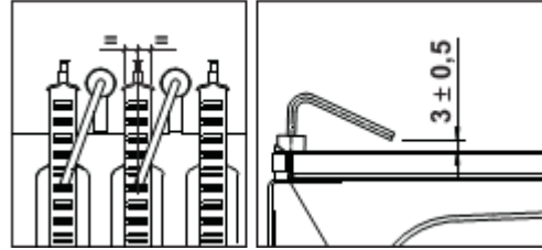
fig. 13 Locatie van de elektroden
