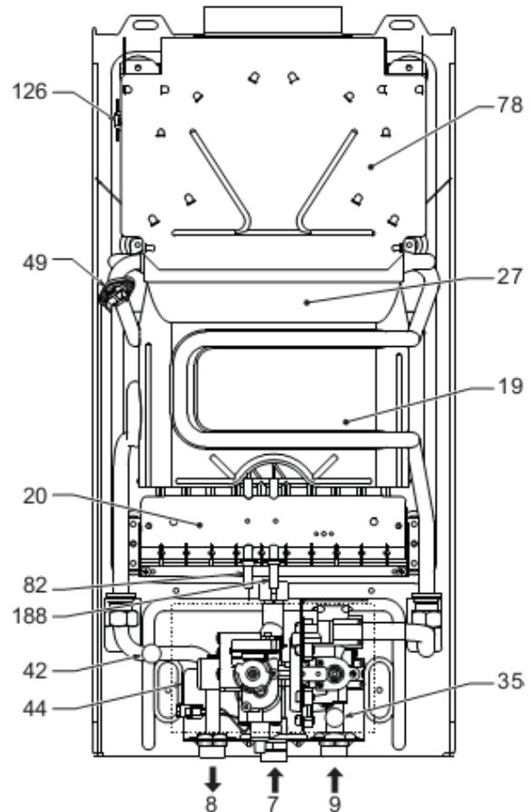
fig. 14 Algemeen overzicht
