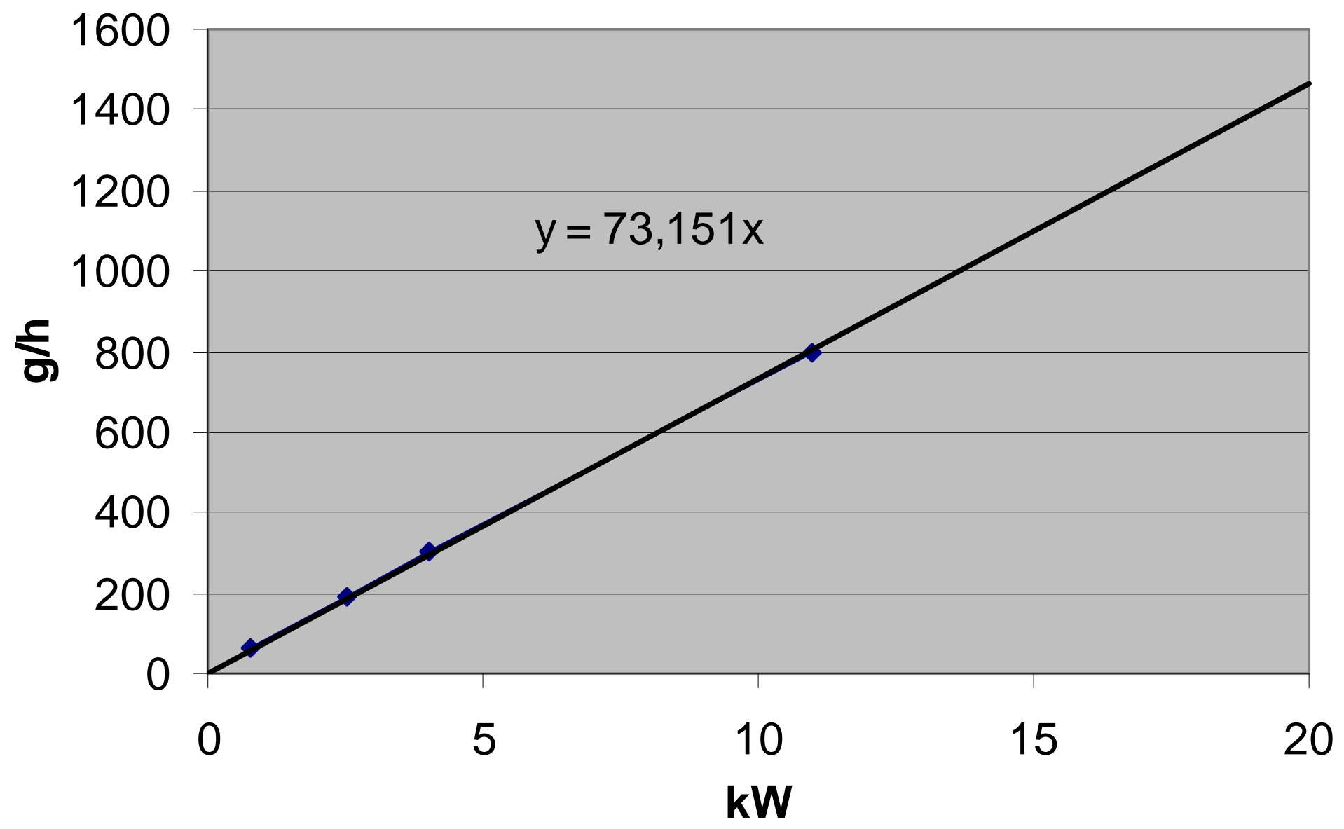
propaan verbruik in gram per uur als functie van kilo Watt
